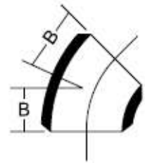
45° Elbow
